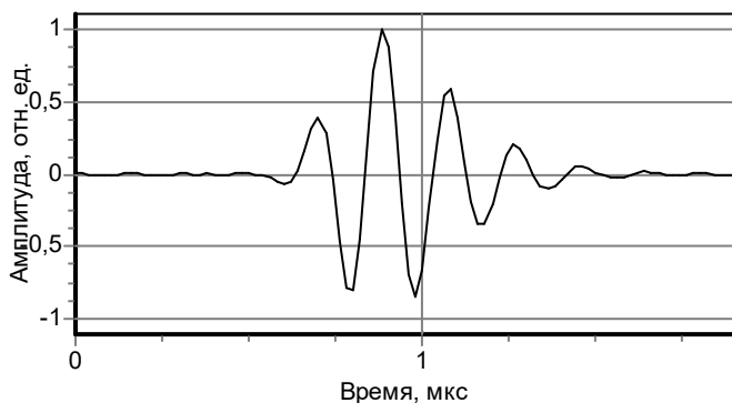
Форма эхосигнала
